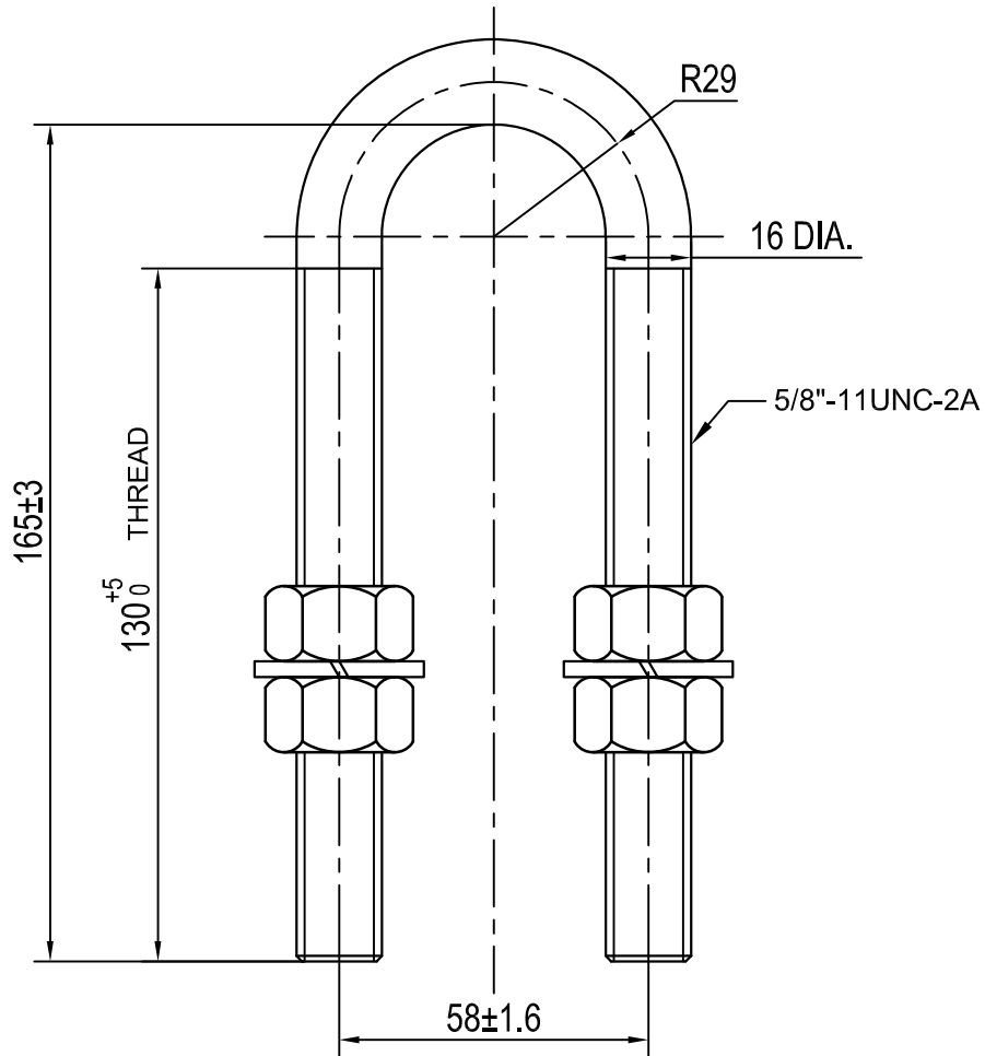
U-BOLT
