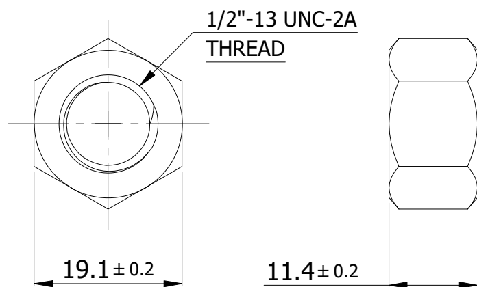
1/2"-13 UNC-2A NUT SS
